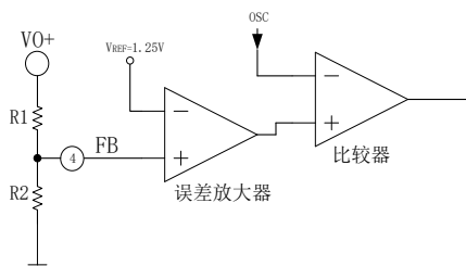
图 8.5 EG1198 输出电压调整电路
